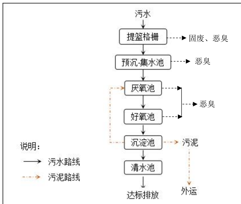
图 5-4 15m³/d 污水处理站工艺流程及产污环节图
