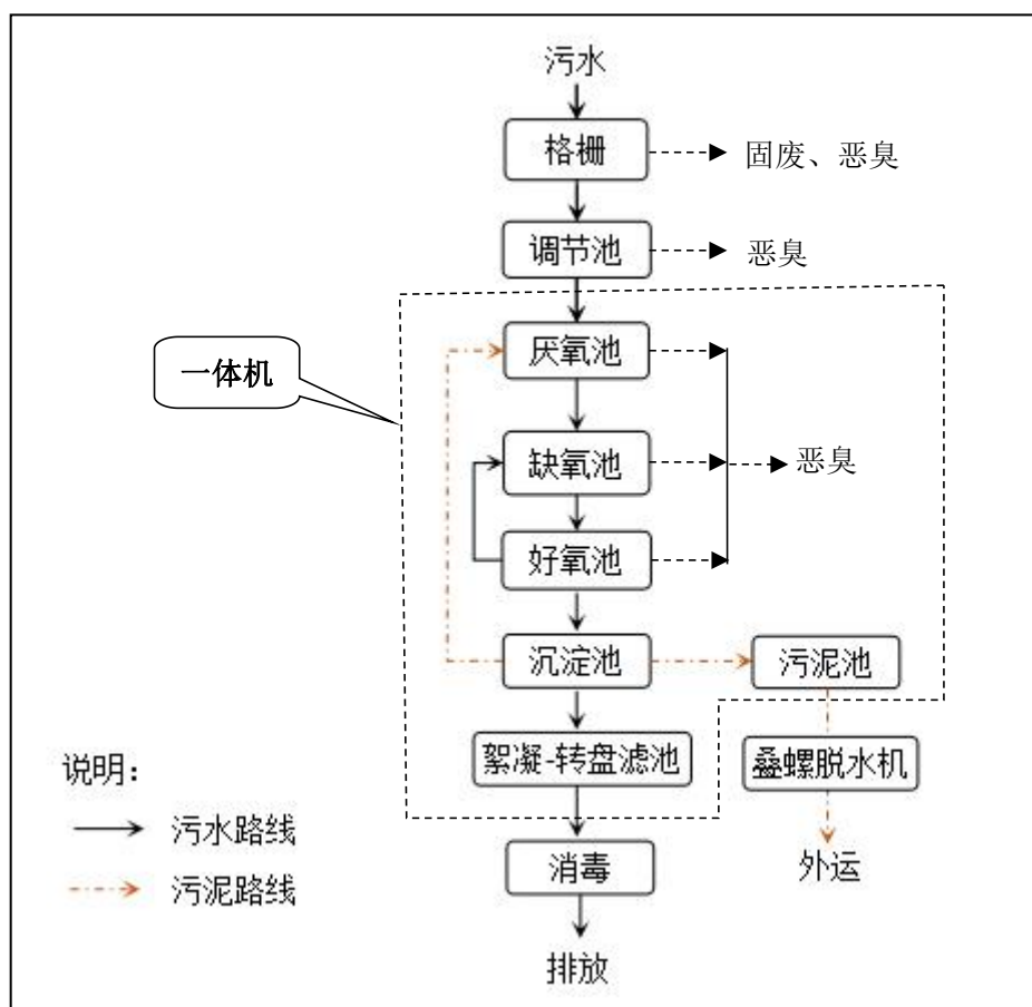
图 5-3 项目 490m 3 /d 桃园村污水处理站生产工艺流程及产污环节图
